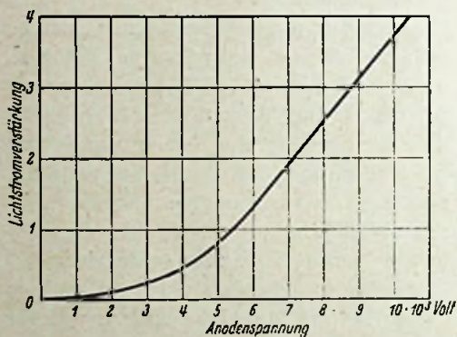
Fig. 5. De verhouding van secundairen tot primairen lichtstroom bij verschillende anodespanningen en bij ongeveer gelijke spectrale intensiteitsverdeling voor kathode en scherm.
