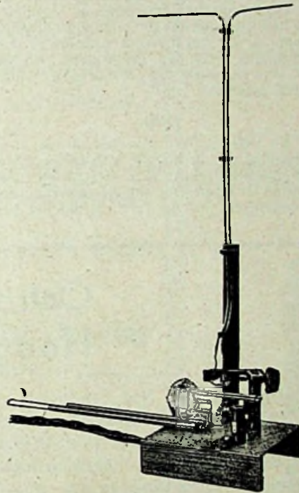
Fig. 2. Typische oscillatorschakeling om met de 316A golven van 60 cm op te wekken.
