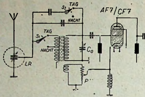
Fig. 2. Principe der bandbreedteregeling (dag- en nachtschakeling) van de „Unix”. Het toestel heeft nog instelbare zeeffkringen (voor lange golf en voor middengolf in de antenne). De eindlamp is hier niet afgebeeld. Men merke de terugkoppeling uit den kathodekring der detectorlamp op.
