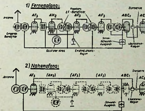
Fig. 7. Hoe de omschakeling super tot 2-krings ontvanger in den 8-lamper „Ultramar 37“ van Körting plaats heeft; menglamp en mf versterker gaan buiten werking; alleen het ingangsbandfilter blijft over. (De nog aanwezige 2de l.f.r. lamp en balansindtrap met twee elkaar aanvullende luidsprekers hebben wij niet afgebeeld).
