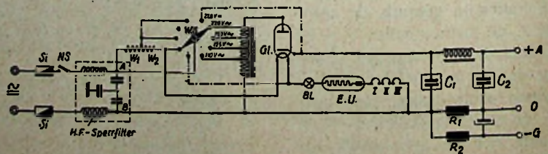
Fig. 4. Schakeling van de voedingsapparatuur der gelijk-wisselstroomtoestellen van Körting, met spaartransformator, die zorgt, dat althans op alle wisselspanningen gelijke praestaties worden verkregen. EU is een ijzer-urdox-weerstand, die de spanning langzaam laat opkomen en daarna den gloeistroom constant houdt.
